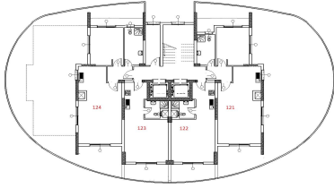
Penthouse Kat Planı
